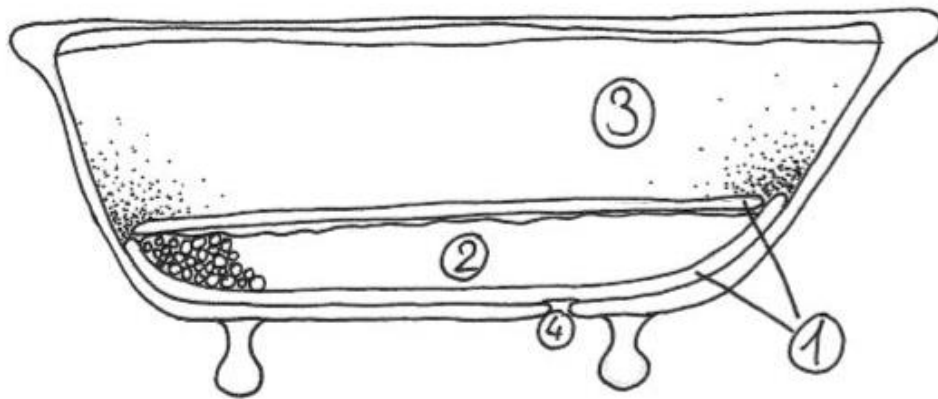
Skizze: Querschnitt Hochbeet aus Badewanne
